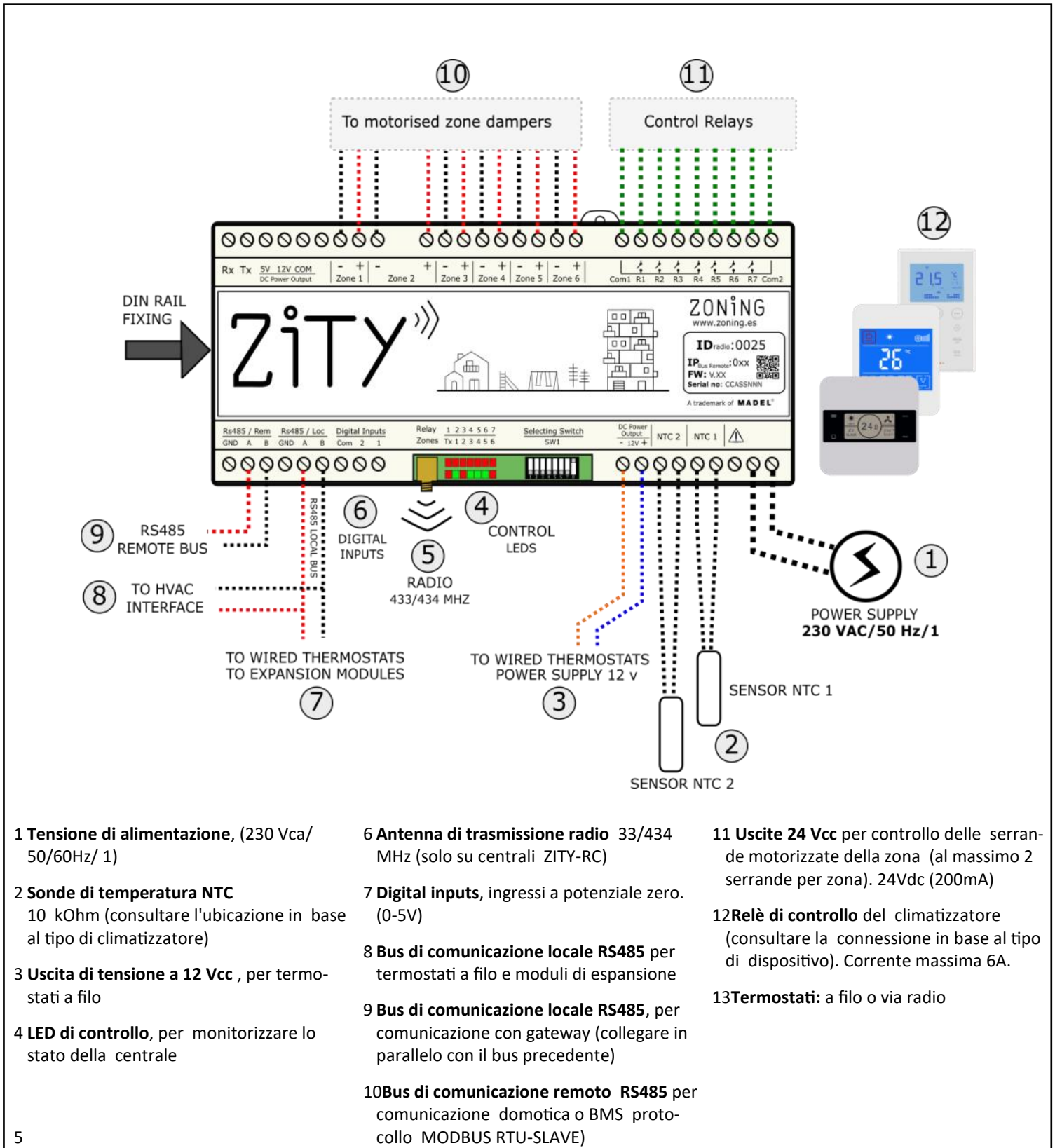
Fig.1 Connessione di tutti i componenti di ZONING SYSTEM nella centrale di controllo ZITY
